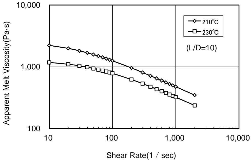
图 1 索阿诺尔™ D2908 的熔融粘度
