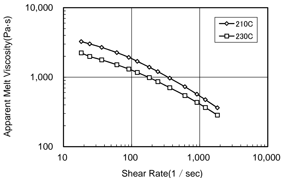
图 1 索阿诺尔™ DT2904RB 的熔融粘度
